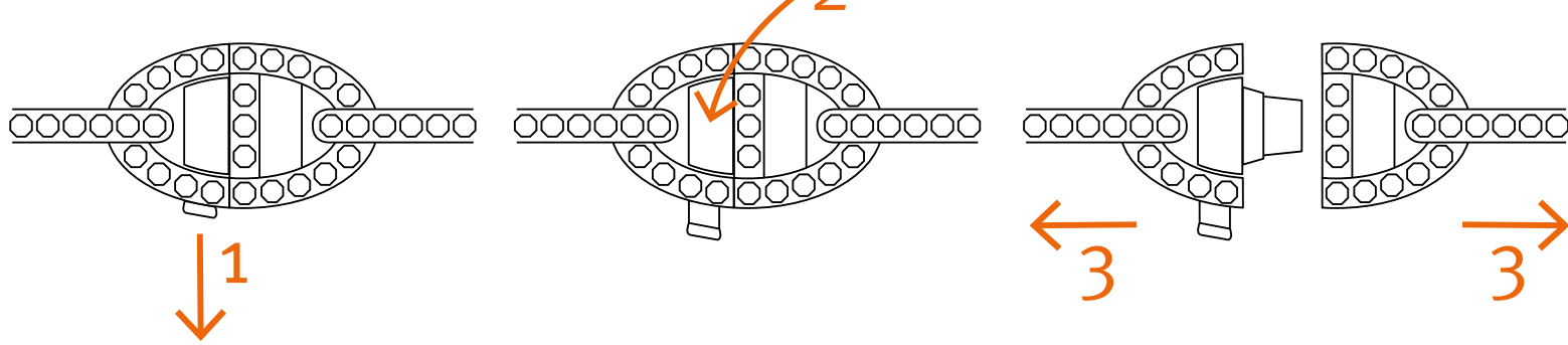
锚链链扣
